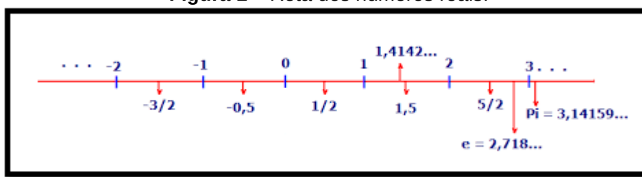
Figura 1 – Reta dos números reais.
